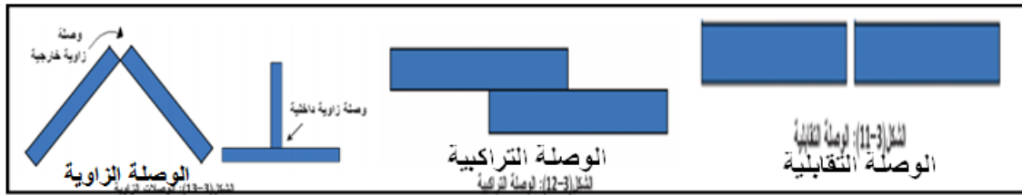
شكل (٣) يوضح أنواع الوصلات اللحامية
